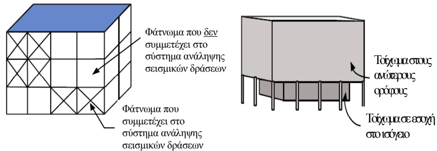
Σχ. Σ5.1 Παραδείγματα μη-κανονικότητας καθύψος: Διακοπή φορέα καθύψος (αριστερά), εκτός επιπέδου εσοχή (δεξιά)
