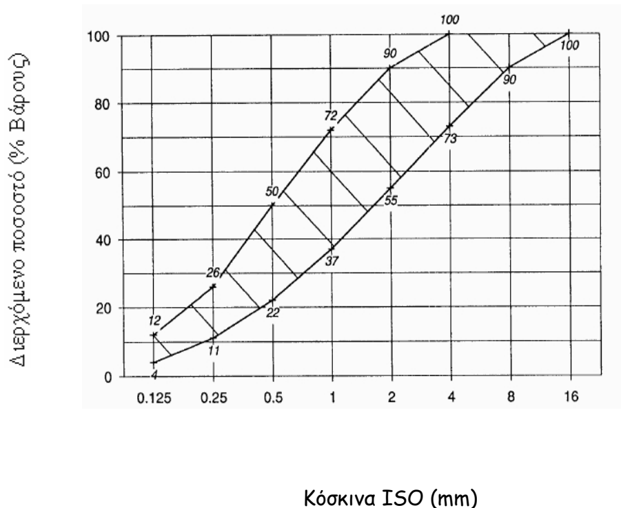
Εικόνα 6: Ορια κοκκομετρικής διαβάθμισης αδρανών για χρήση σε εκτοξευόμενο σκυρόδεμα, [3]
