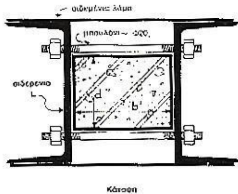
Σχήμα 5: Διάταξη μορφοσίδερου
