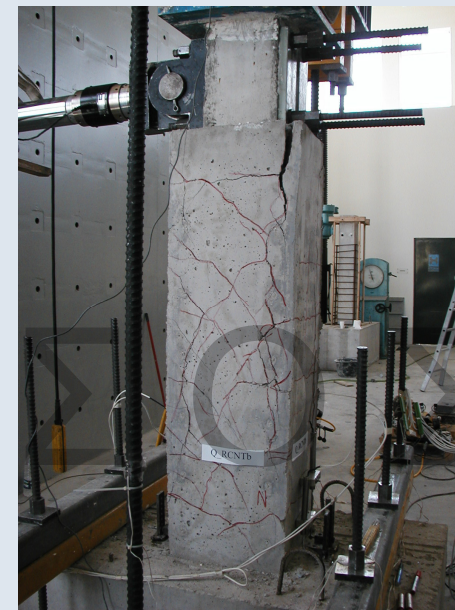
Βλάβες σε Δοκίμιο με Έγχυτο Σκυρόδεμα, Λεία Διεπιφάνεια χωρίς Διατηρητικούς Συνδέσμους 50
