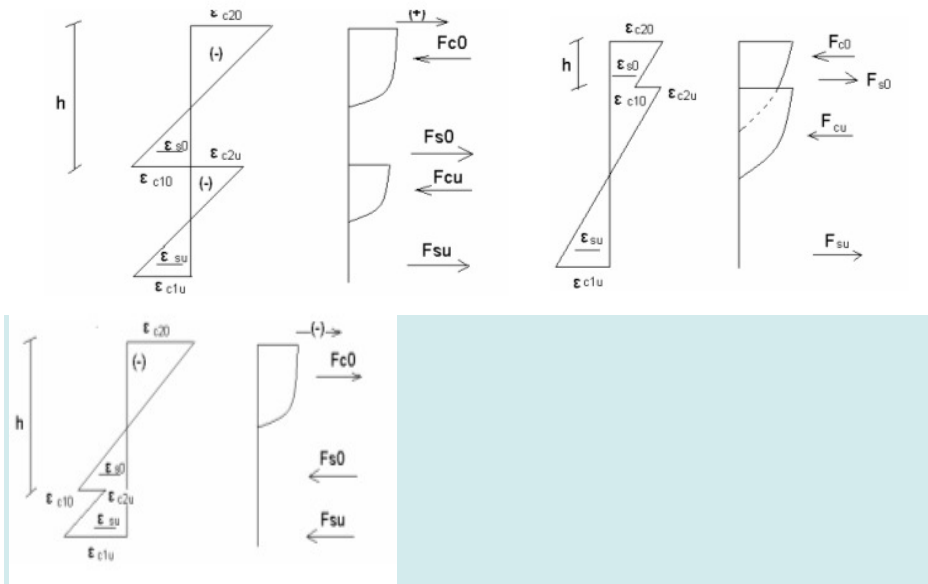
Πιθανή Κατανομή Παραμορφώσεων και Τάσεων
